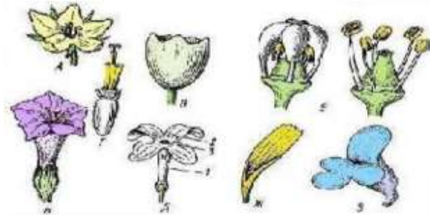
Рис. 22 Формы сростнолепестных венчиков - колесовидный (вербейник Lysimachia vulgaris ) Б - воронковидный (табак Nicotiana tabacum )
