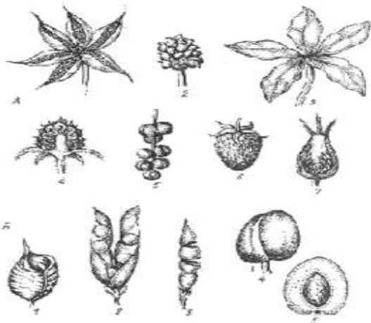
Рис. 31 Типы апокарпных плодов А - сухие и сочные апокарпии:
