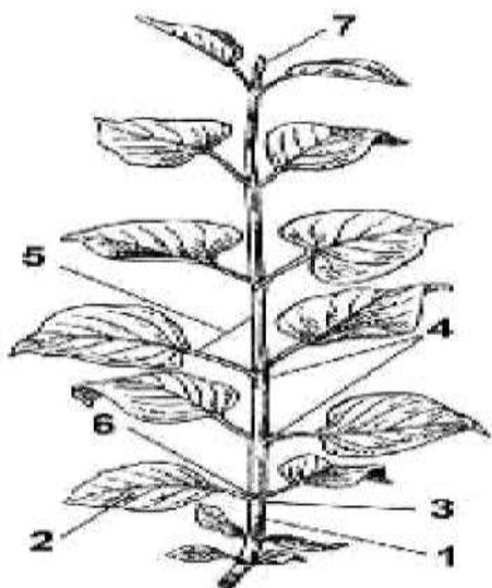
Рис. 5 Строение побега 1 - верхушечная почка 2 - пазушная почка 3 - междоузлие 4 - узел 5 - пазуха листа 6 - лист 7 - стебель
