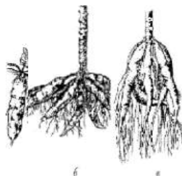
Рис. 2 Виды корневых шишек а- батат; б- маниока; в- георгина
